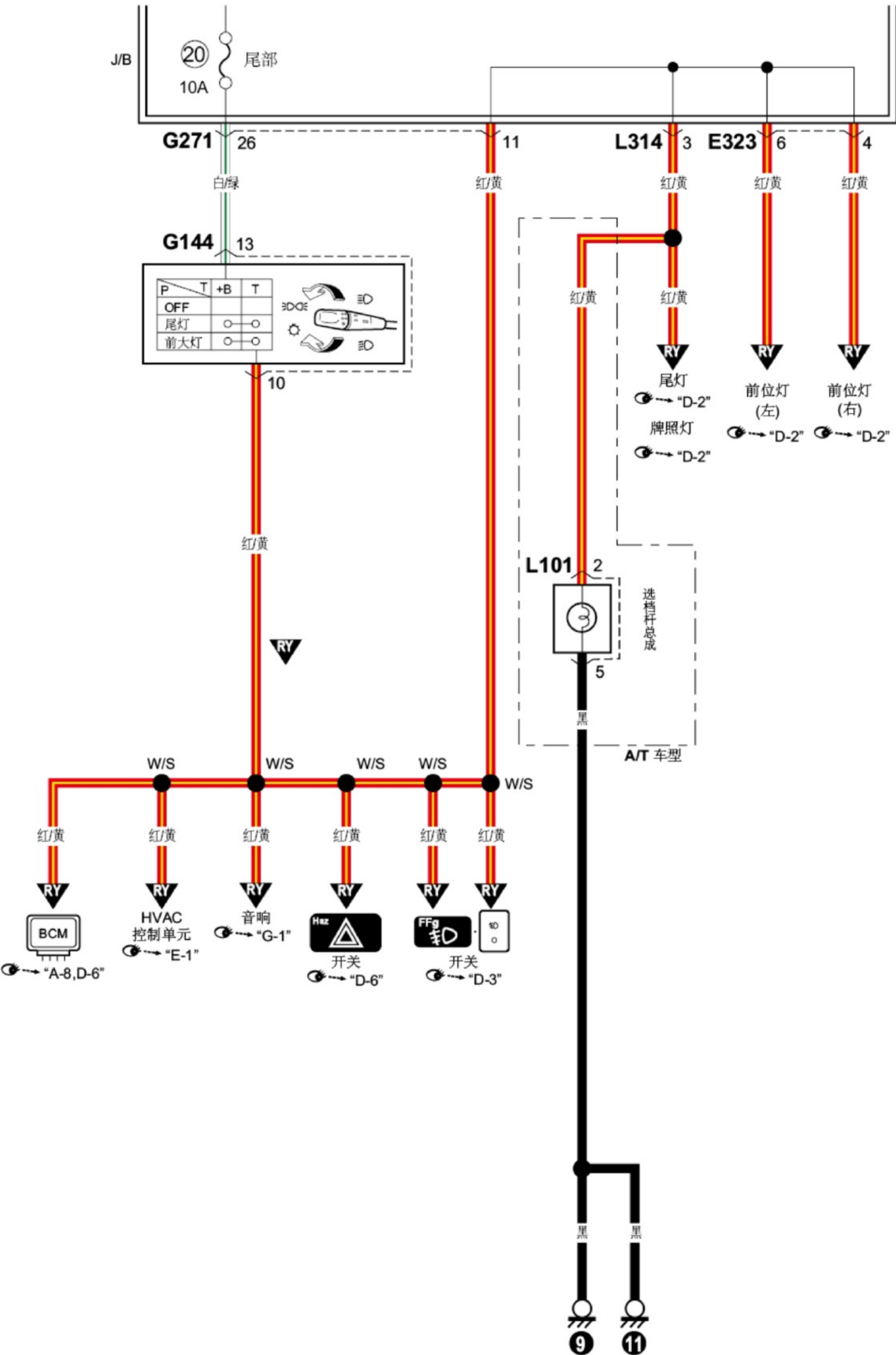
D-4照明灯系统电路图
